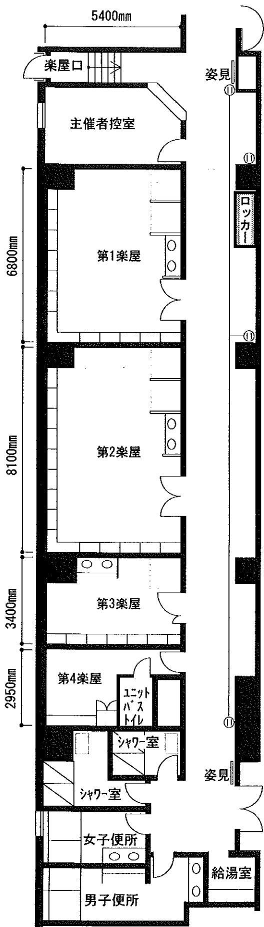
大ホール楽屋 1/150
