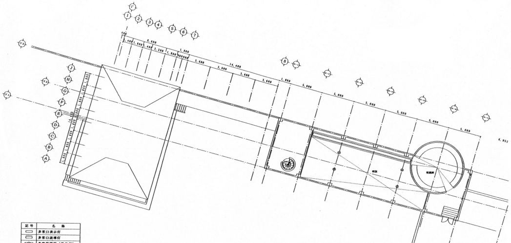
物見塔レベル平面図
